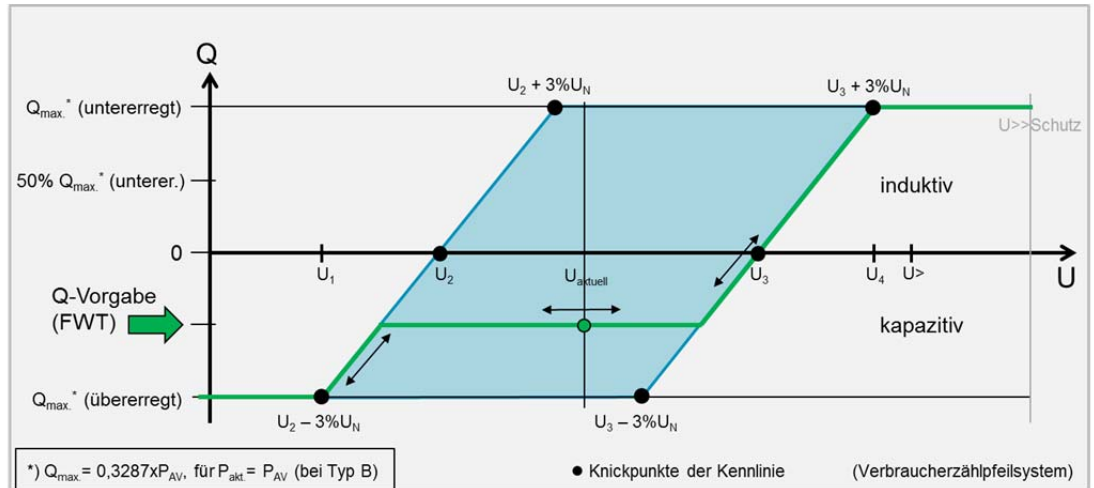
Bild 2.6: Q(U)-Verhalten für eine EZA vom Typ A bei Q-Soll = 0,5 x 0,3287 x P AV kapazitiv (übererregt)
