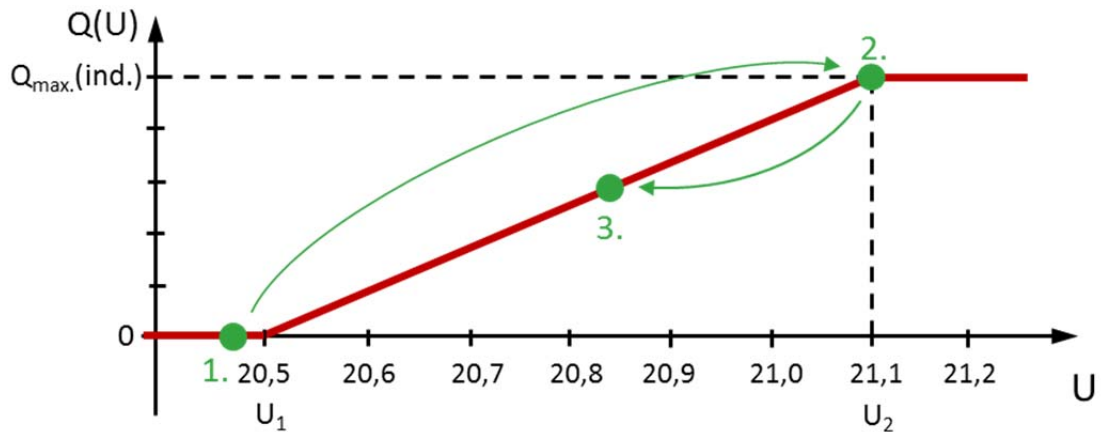
Bild 8.2: Q(U) -Kennlinie für Testsystem
