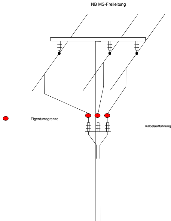
Bild 7.2: Eigentumsabgrenzen bei einer Kabelaufführung am Mast einer MS-Freileitung
