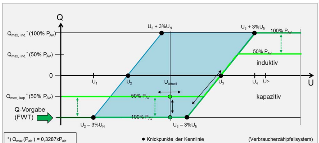
Bild 2.8: Q(U)-Verhalten für eine EZA vom Typ B bei Q-Vorgabe von 0,3287 \times P_{AV} kapazitiv (übererregt) und P_{akt.} = 50\% P_{AV} (hellgrüne Linie) sowie P_{akt.} = 100\% P_{AV} (dunkelgrüne Linie)
