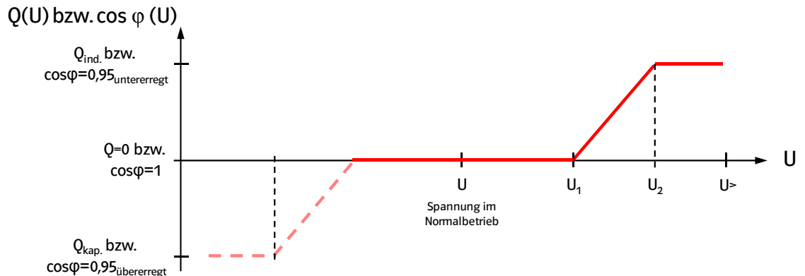
Bild 9.1: Qualitative Darstellung des spannungsabhängigen Blindleistungsverhaltens von Erzeugungsanlagen
