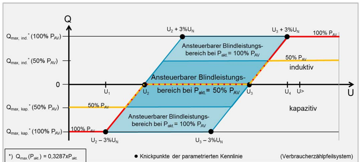
Bild 2.5: EZA vom Typ B: Q(U)-Verhalten (orange) bei P_{akt.}=50\%P_{AV} und Q\text{-Soll}=0 sowie der ansteuerbare Blindleistungsbereich (dunkelblau) für Q\text{-Soll} \neq 0 ; Q(U)-Verhalten (rot) bei P_{akt.}=100\%P_{AV} und Q\text{-Soll}=0 sowie der ansteuerbare Blindleistungsbereich (hell- und dunkelblau) bei Q\text{-Soll} \neq 0
